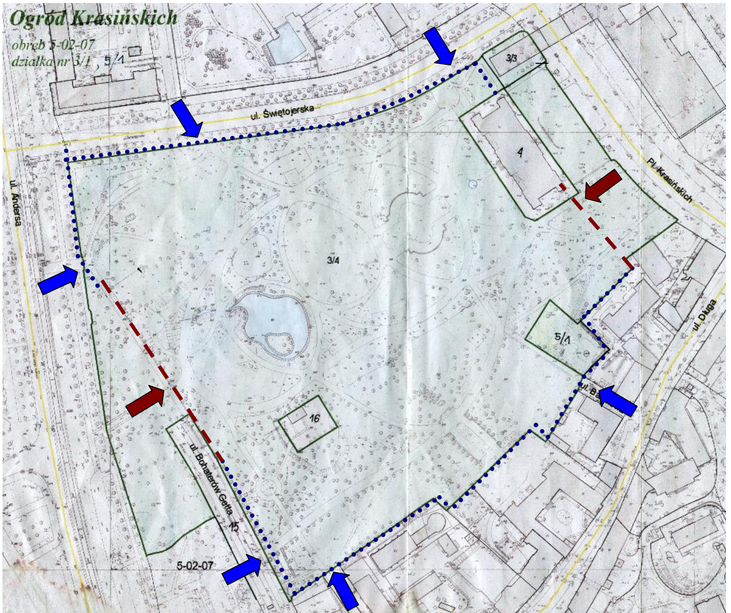
Rys. 8. Proponowany przebieg ogrodzenia Ogródu Krasińskich w Warszawie
