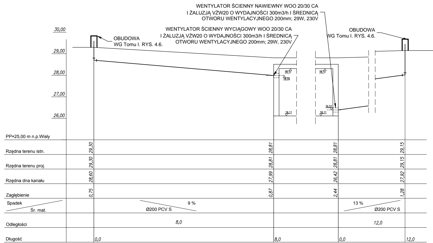
WENTYLACJA MECHANICZNA POMIESZCZENIA TECHNICZNEGO STAWU
